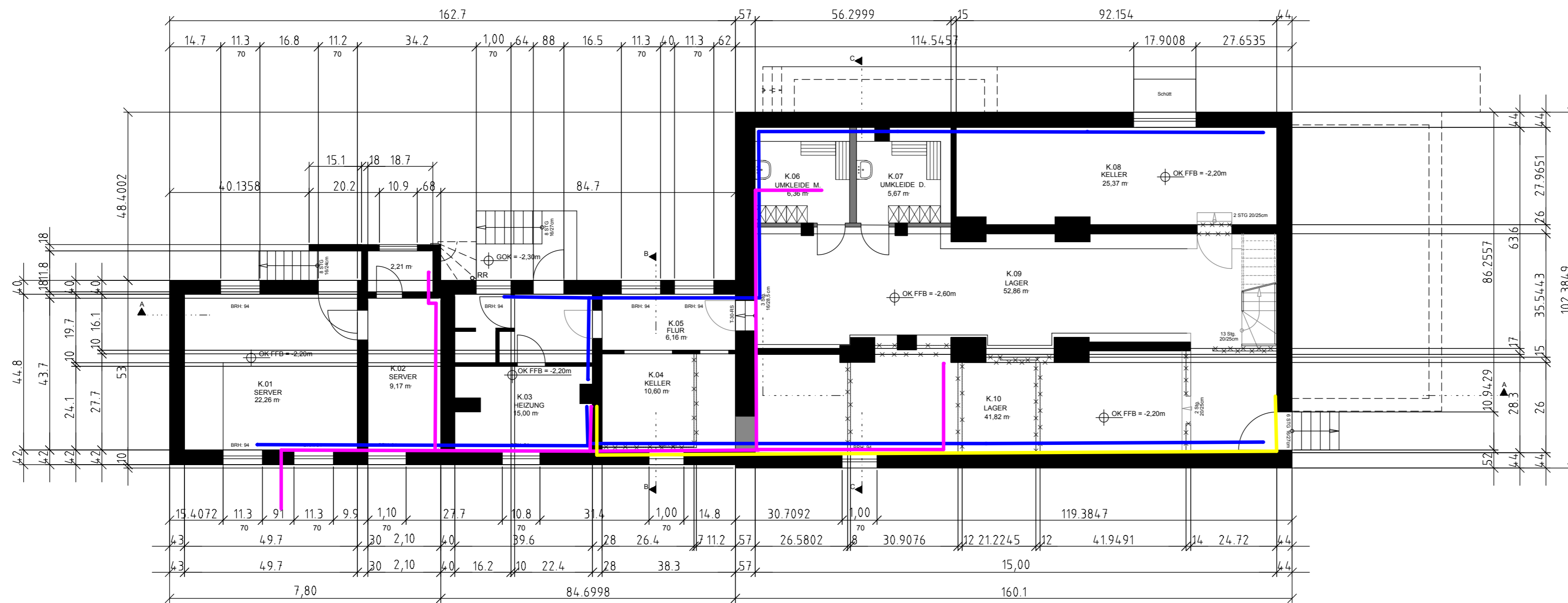
UNTERGESCHOSS
