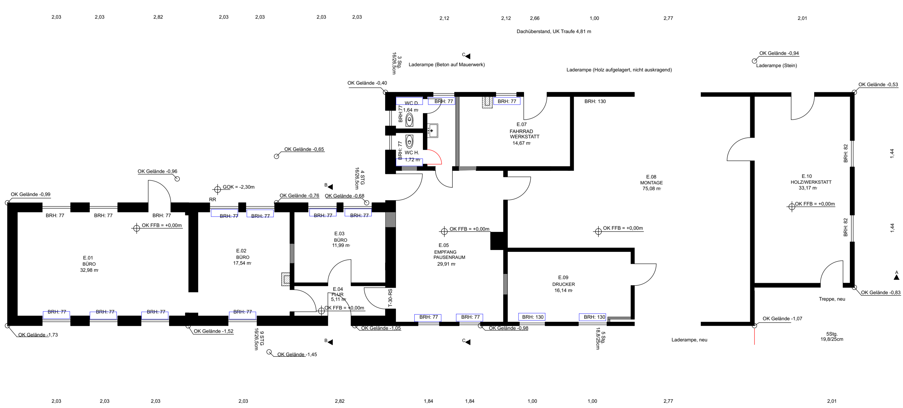
EDGESCHOSS
