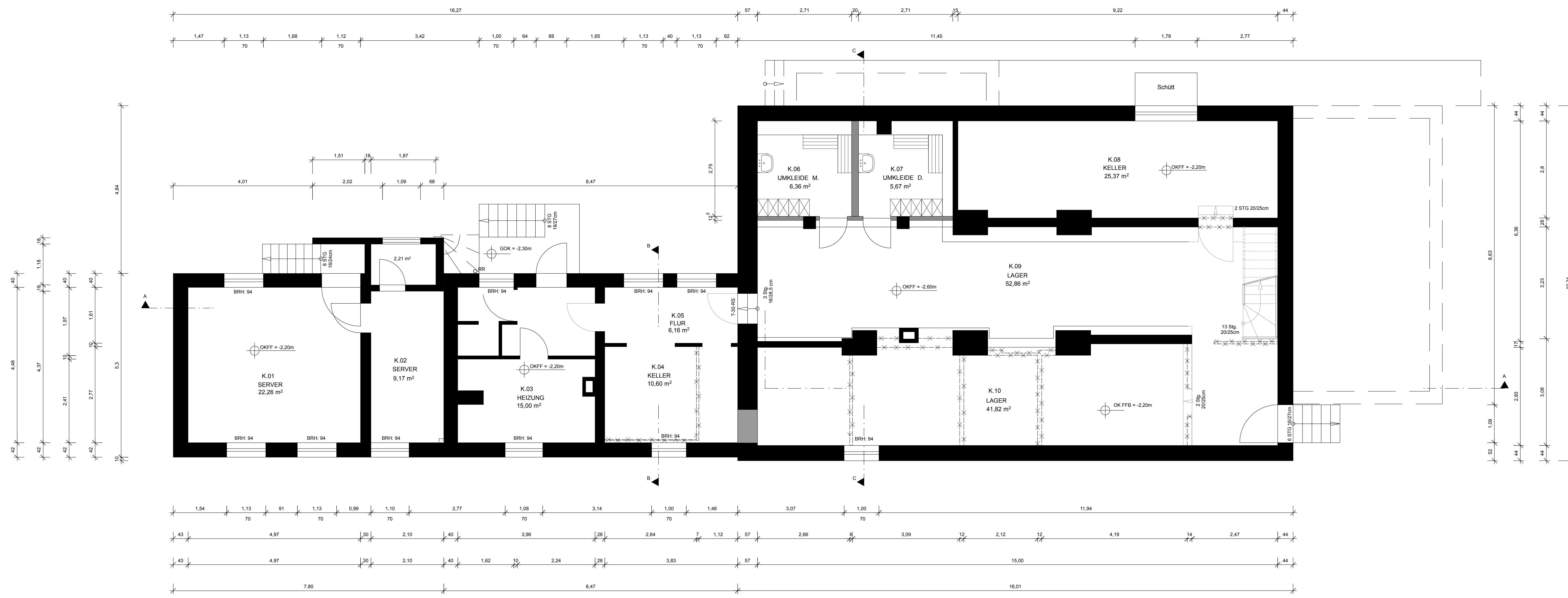
UNTERGESCHOSS
